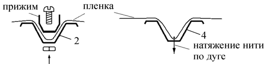
Рис.8 Крепление плёнки прижимами и нитью
