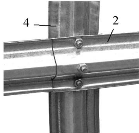
Рис.5 Узел Б Вид изнутри
